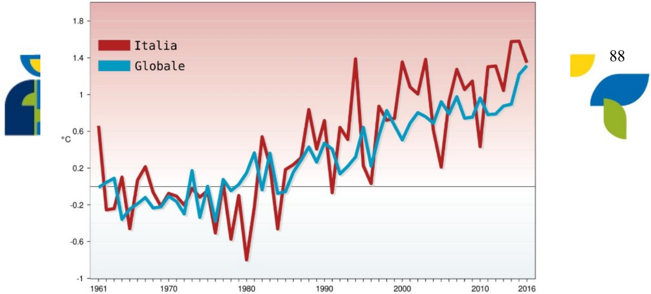
Serie delle anomalie di temperatura media globale sulla terraferma e in Italia, rispetto ai valori climatologici normali 1961 - 1990. Fonti: NCDC/NOAA e ISPRA. Elaborazione: ISPRA
